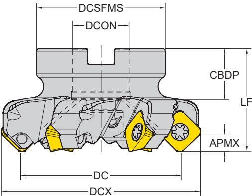
<S> Торцово-цилиндрическая фреза
