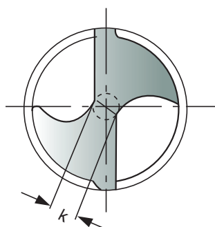
Рис. 1. Толщина перемычки k
