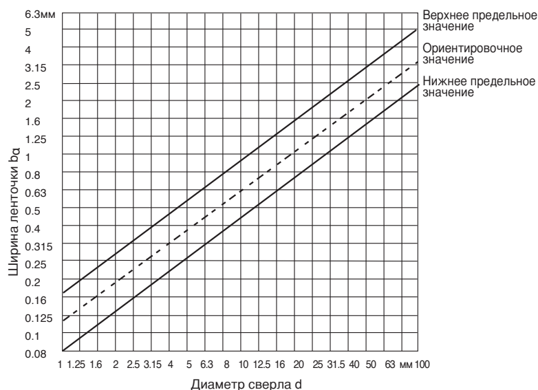
Рис.4. Ширина ленточки b_{\alpha}
