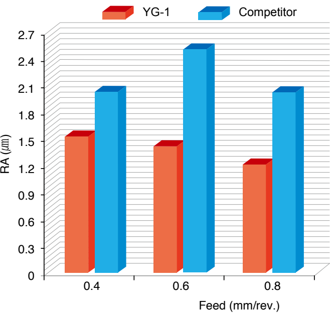
Шероховатость обработанной поверхности
