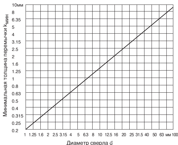
Рис.2. Толщина перемычки k_{\min}
